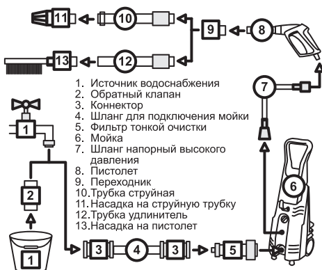
Рис. 13 Схема подключения аппарата с дополнительным оборудованием
