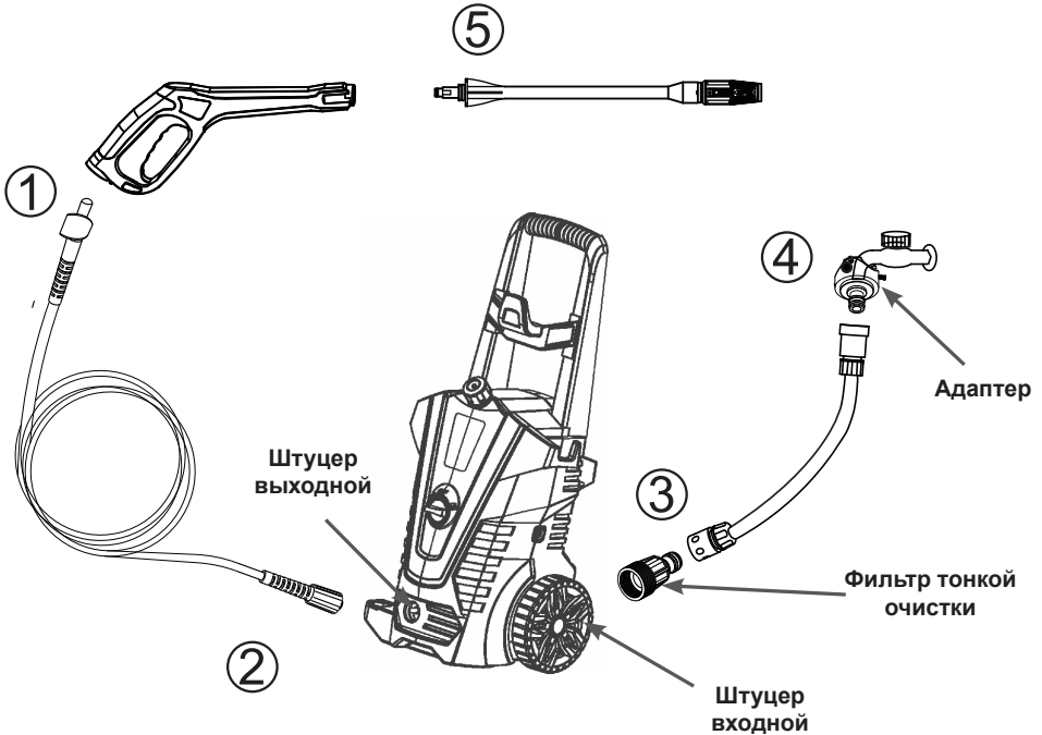
Рис. 2 Сборка аппарата
